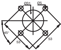
Door drilling for OH_ handles
